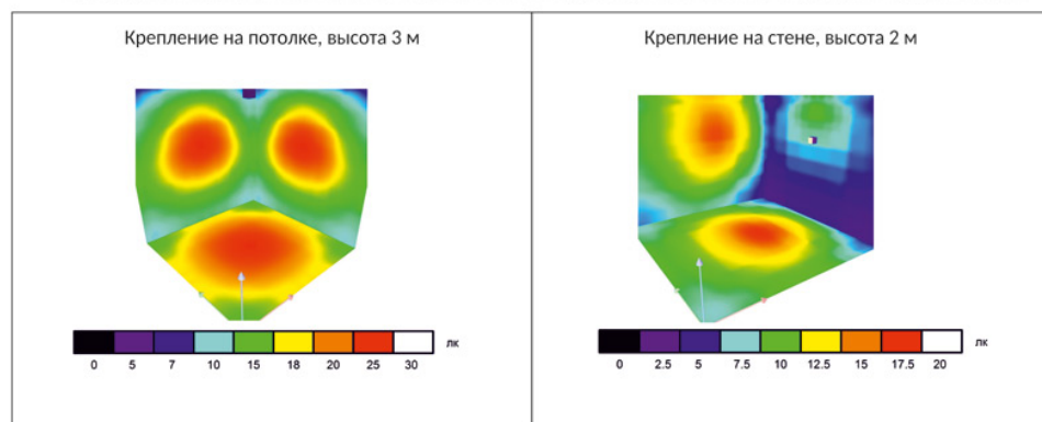
Распределение освещенности в зависимости от высоты подвеса для светильника с прозрачным рассеивателем
